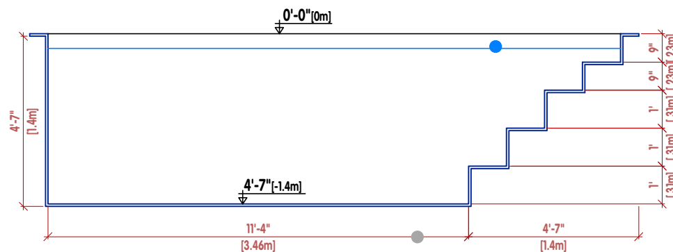
CORTE LONGITUDINAL
