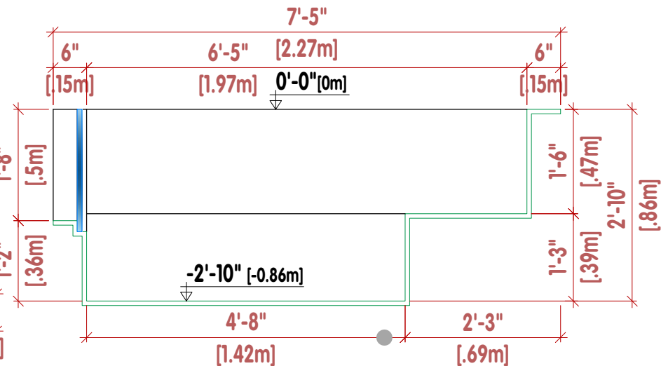
CORTE TRANSVERSAL | CROSS SECTION | LA COUPE TRANSVERSALE
